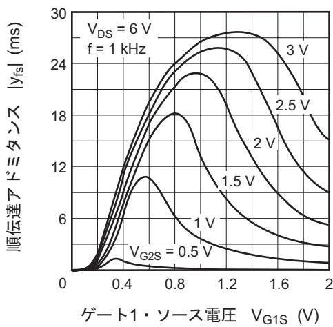
順伝達アドミタンス対 ゲート1・ソース電圧特性
