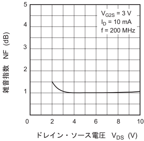
雑音指数対ドレイン・ソース電圧特性
