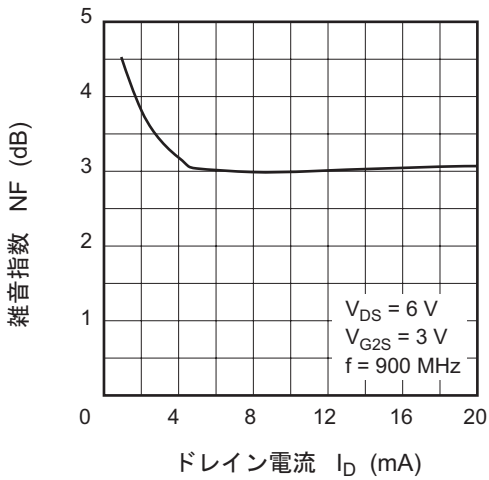
雑音指数対ドレイン電流特性
