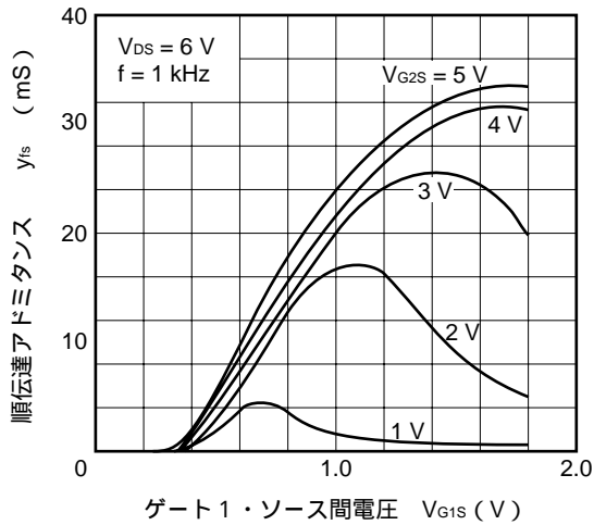
順伝達アドミタンス vs. ゲート1・ソース間電圧
