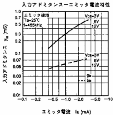
エミッタ接地, 455kHz yパラメータ
