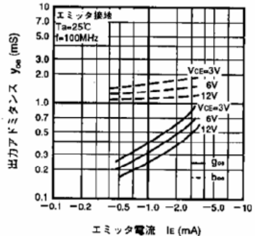
出力アドミタンス-エミッタ電流特性
