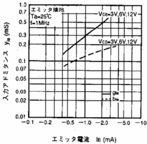
入力アドミタンス-エミッタ電流特性
