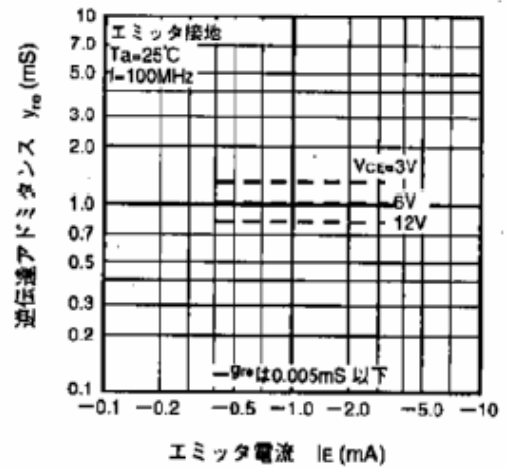
逆伝達アドミタンス-エミッタ電流特性
