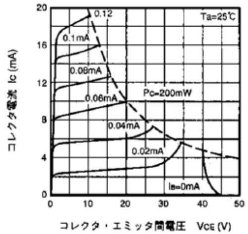
エミッタ接地出力特性 (2)
