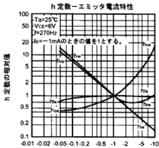
エミッタ接地h定数(標準値)
