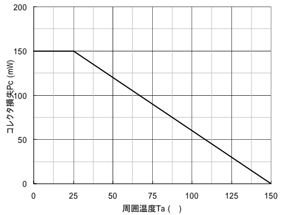
コレクタ損失 - 周囲温度特性
