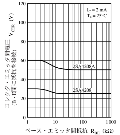
V_{CER} - R_{BE}
