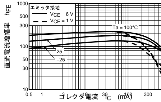
h_{FE} - I_C
