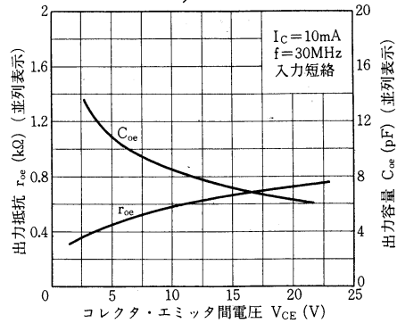
2SC32 r_{oe}, C_{oe}-V_{CE} 特性
