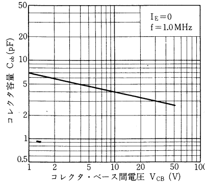
C_{ob}-V_{CB} 特性
