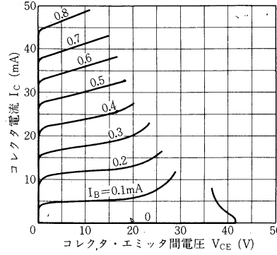
2SC32 I_c-V_{CE} 特性
