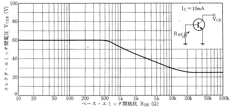
V_{CER}-R_{BE} 特性
