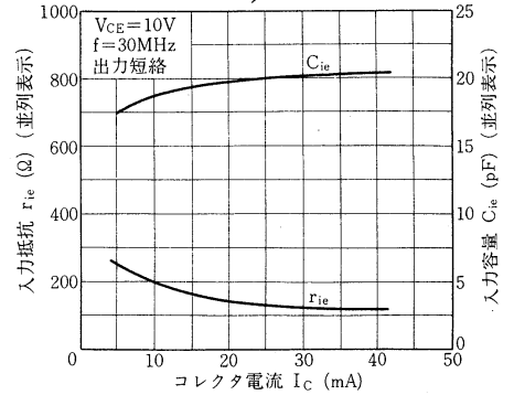
2SC32 r_{ie}, C_{ie}-I_C 特性
