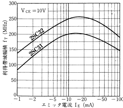
f_T-I_E 特性
