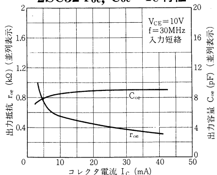
2SC32 r_{oe}, C_{oe}-I_C 特性
