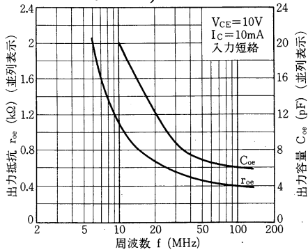
2SC32 r_{oe}, C_{oe}-f 特性
