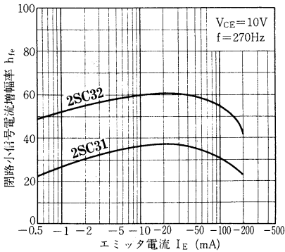
h_{fe}-I_E 特性
