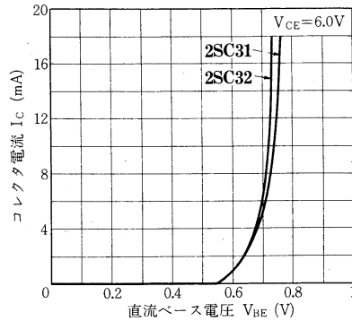
I_c-V_{BE} 特性
