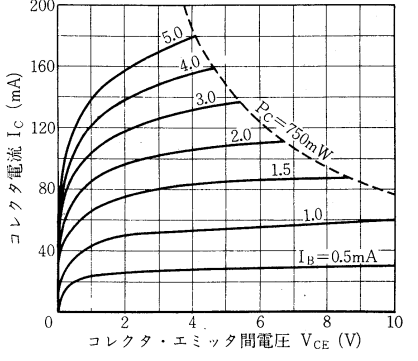
2SC32 I_c-V_{CE} 特性
