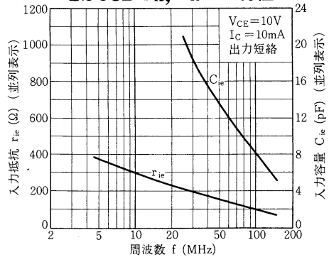
2SC32 r_{ie}, C_{ie}-f 特性
