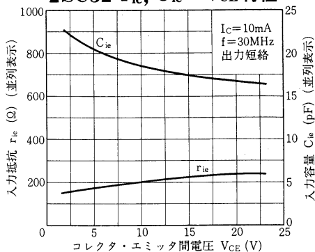
2SC32 r_{ie}, C_{ie}-V_{CE} 特性
