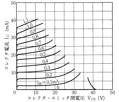
2SC31 I_c-V_{CE} 特性
