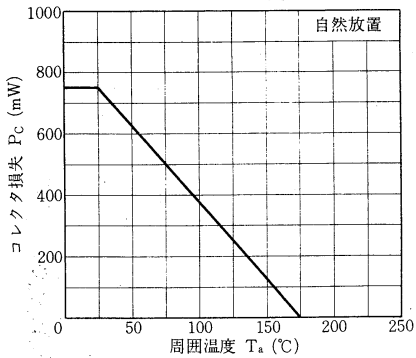
P_c-T_a 特性
