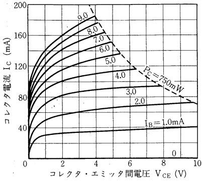
2SC31 I_c-V_{CE} 特性
