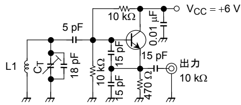
L1: \phi 0.8 \text{ mm} 銀メッキ銅線 3 回巻, 内径 \phi 10 \text{ mm} 長さ 10 mm
