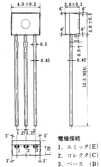
外形図 (単位: mm)
