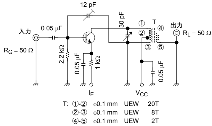
図1 電力利得測定回路
