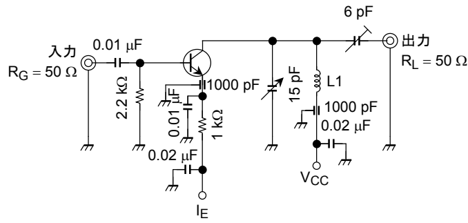
L1: φ0.8 mm 銀メッキ銅線 (空心 4T, 巻径 10 mm, 巻長 8 mm)
