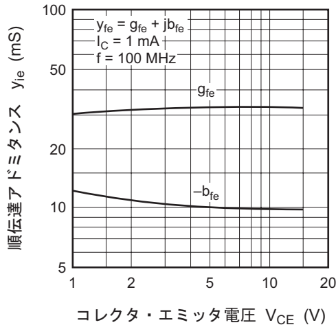
順伝達アドミタンス対 コレクタ・エミッタ電圧特性
