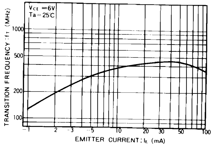
Fig.10 利得帯域幅積-エミッタ電流特性
