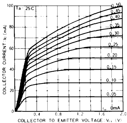
Fig.3 エミッタ接地出力静特性 (I)
