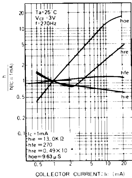
Fig.13 h定数—コレクタ電流特性
